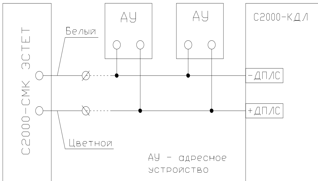
Рисунок 2.2.4.1 Схема подключения
