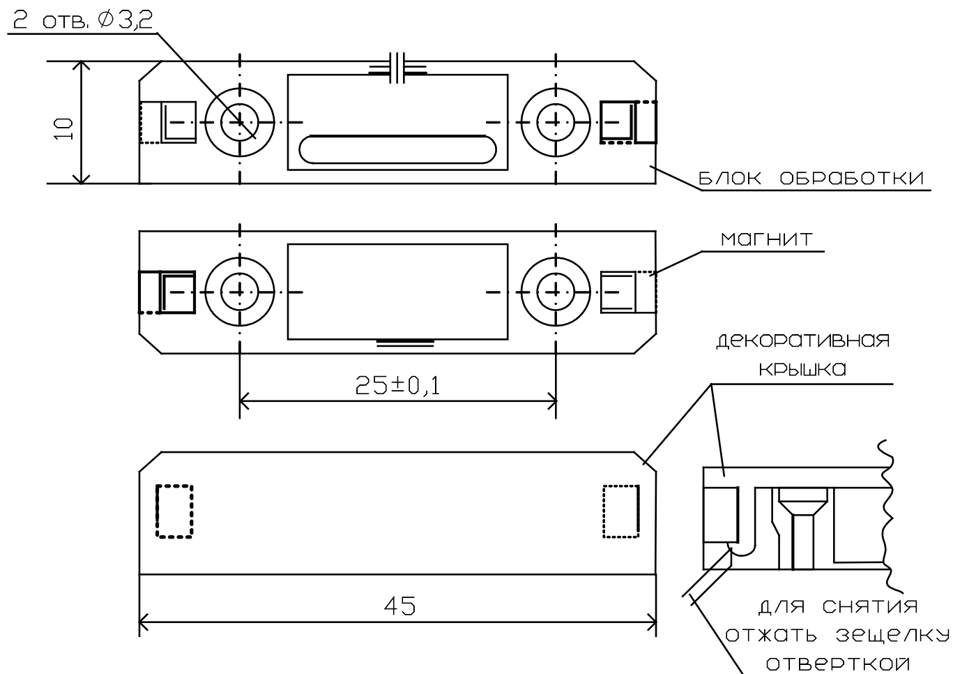
Рисунок 2.2.3.1 Установочные размеры
