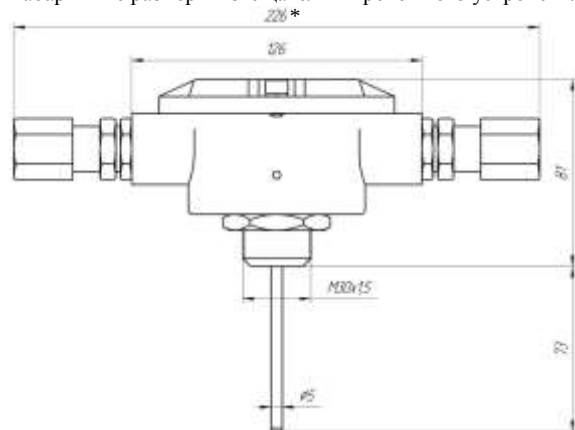
* - зависит от типа используемых кабельных вводов Рисунок 1 – Габаритные размеры извещателя
