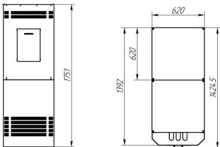
Сборка стеллажа СА-20-250 (М) с секцией на узкой стороне
