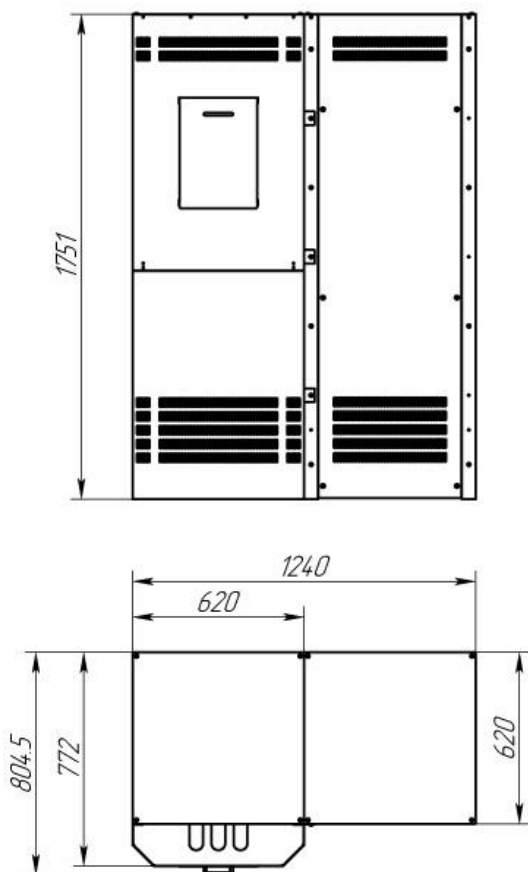
Сборка стеллажа СА-20-250 (М) с секцией на широкой стороне
