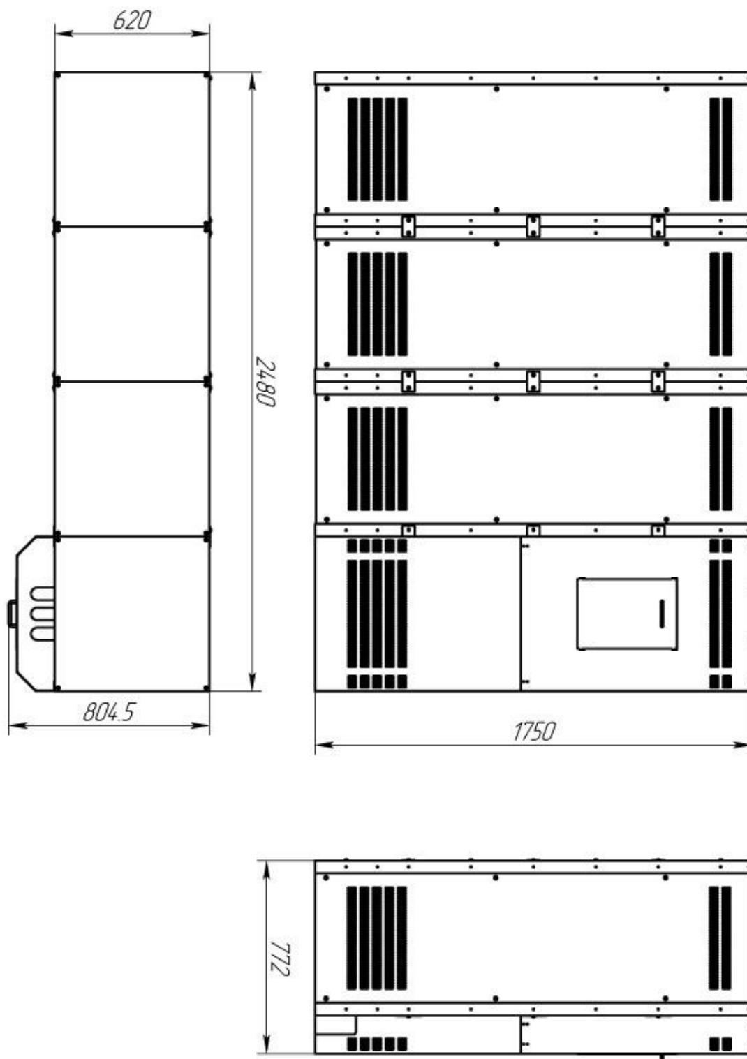
Сборка стеллажа СА-40-250 (М) с секцией на широкой стороне
