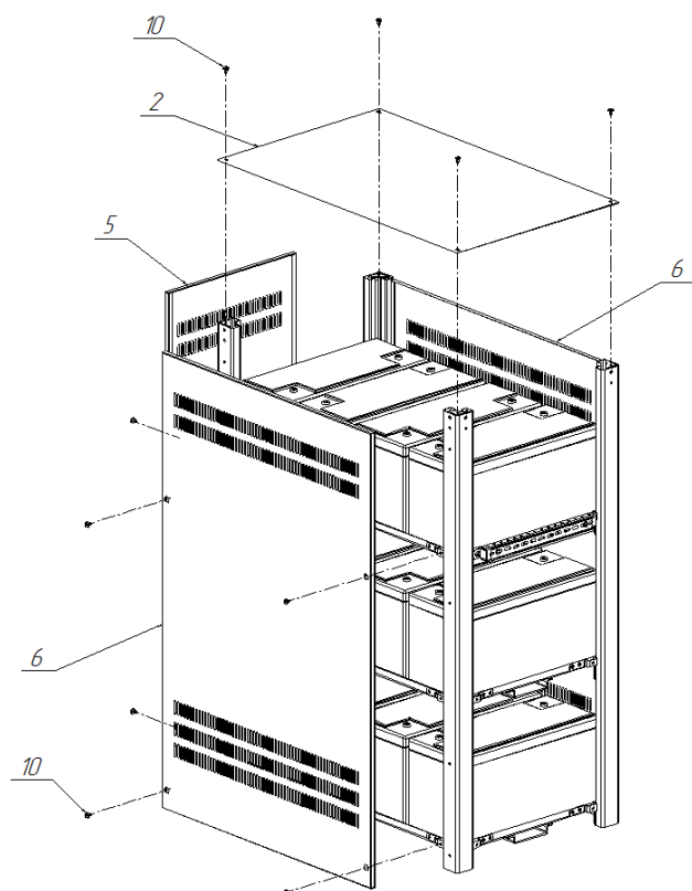
Рис. 6. Установка стенок и крыши
