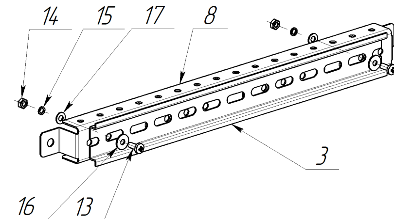
Рис. 4. Установка рейки на кронштейн
