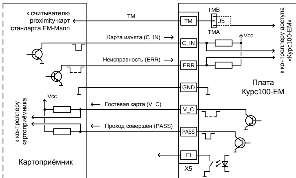
Рис.5 Схема подключения картоприёмника к плате «Курс100-ЕМ» турникета
