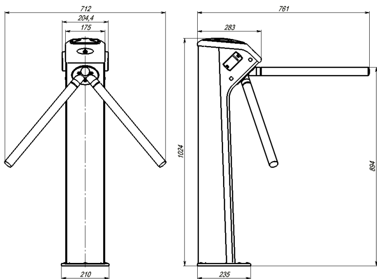
Рис.7Б1 Турникет SA320. Габаритные размеры
