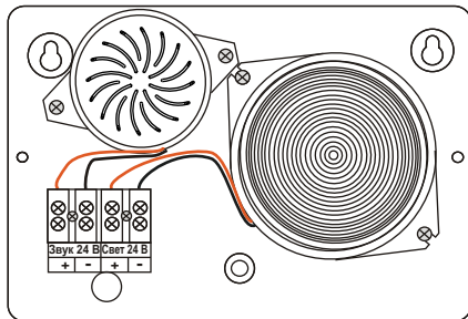
Рис.2 Схема подключения оповещателя.
