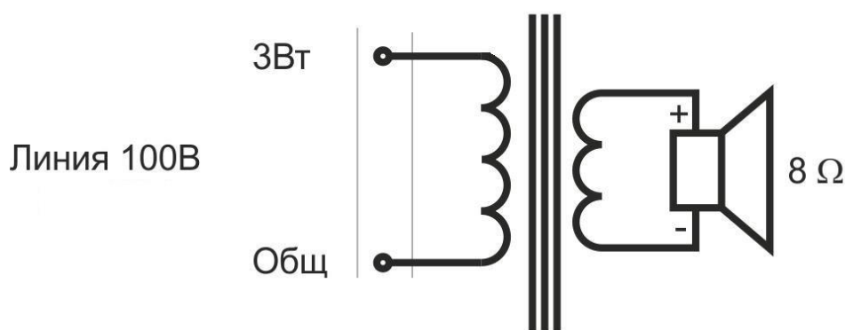
Рис. 2. Схема подключения громкоговорителя.
