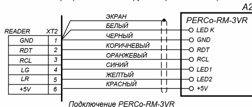
Рисунок 3. Схема подключения со считывателями PERCo-RMC01, PERCo-RM-3VR
