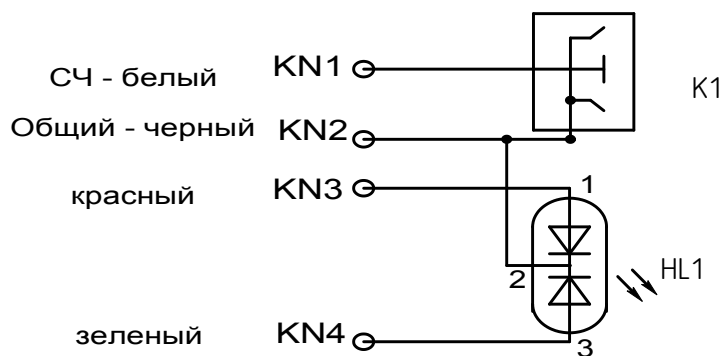
Схема подключения.
