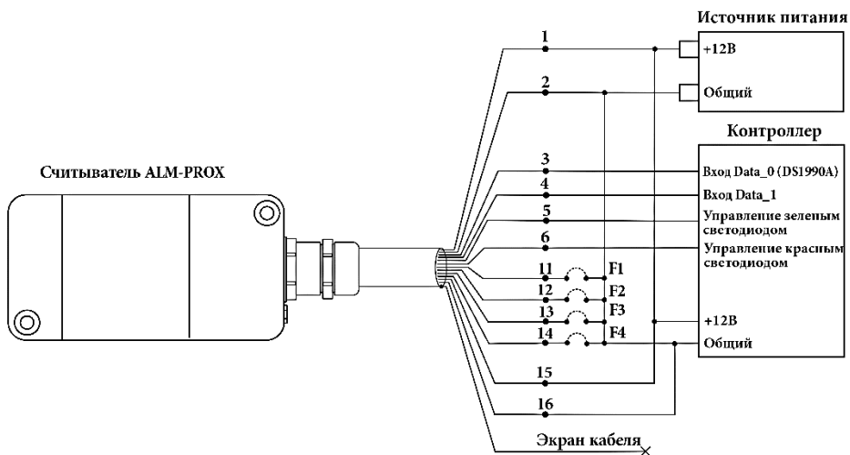
Рисунок 6 - Схема подключения считывателя ALM-PROX к контроллеру СКУД с питанием считывателя от одного источника питания.
