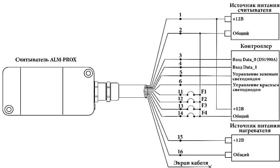
Рисунок 5 - Схема подключения считывателя ALM-PROX к контроллеру СКУД с питанием считывателя от двух источников питания.
