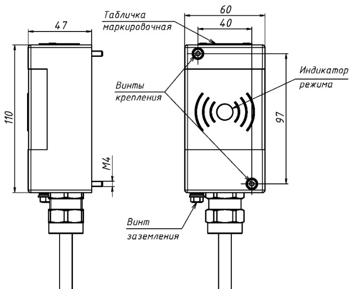
Рисунок 1 - Габаритно-установочные размеры считывателя
