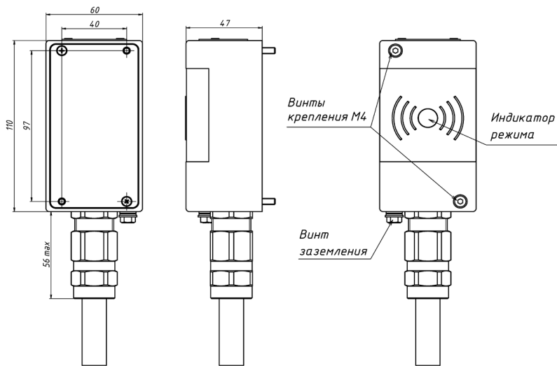
Рисунок 1 - Габаритно-установочные размеры считывателя ALM-RD-S06
