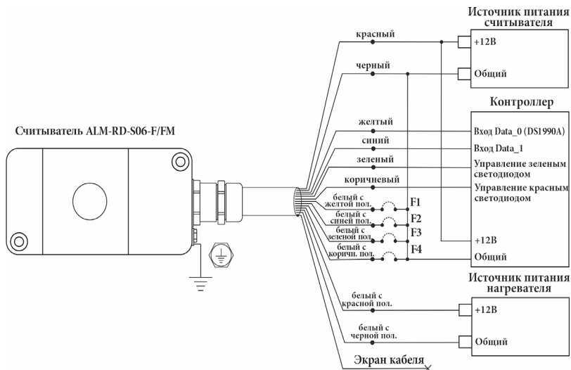
Рисунок 3 – Схема подключения счетчика ALM-RD-S06-F/FM к контроллеру СКУД с разделным питанием счетчика и нагревателя
