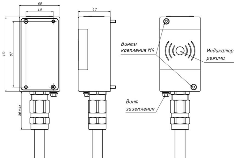
Рисунок 1 - Габаритно-установочные размеры считывателя ALM-RD-S06
