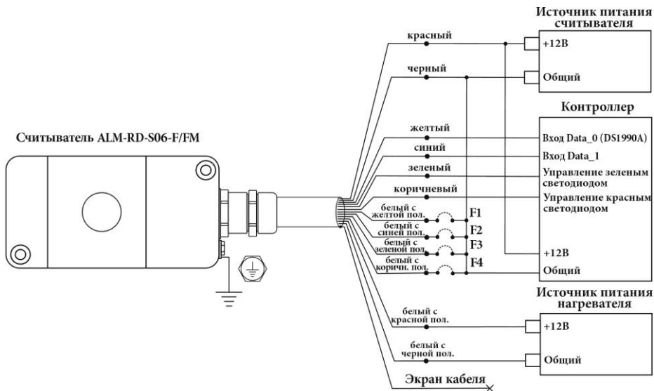
Рисунок 3 – Схема подключения считывателя ALM-RD-S06-F/FM к контроллеру СКУД с раздельным питанием считывателя и нагревателя
