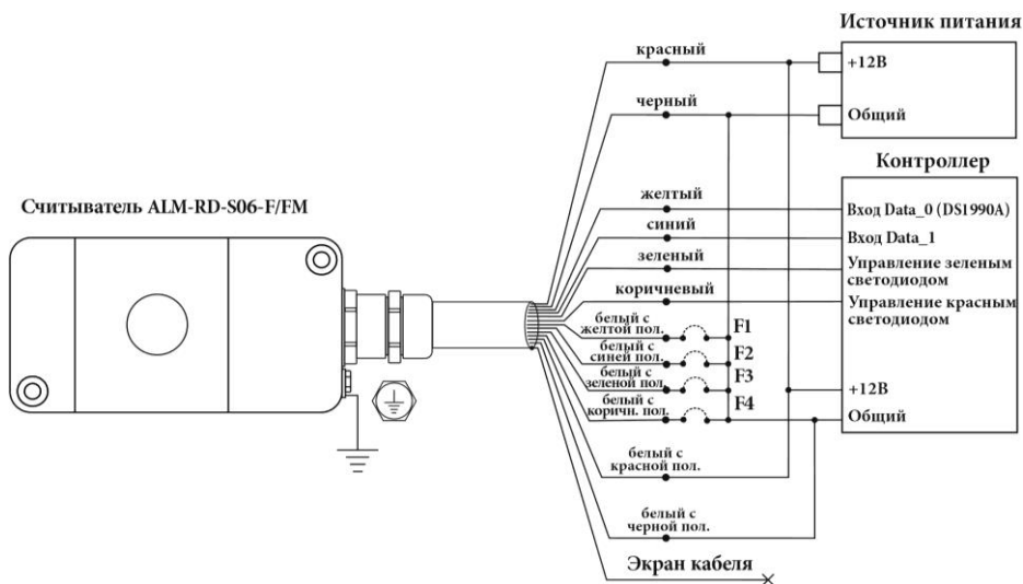
Рисунок 4 – Схема подключения считывателя ALM-RD-S06-F/FM к контроллеру СКУД с питанием считывателя и нагревателя от одного источника питания.
