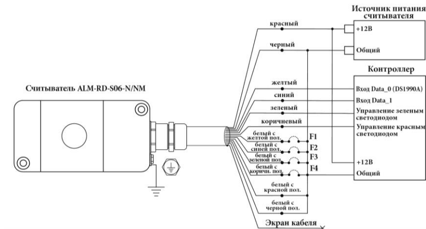
Рисунок 2 – Схема подключения считывателя ALM-RD-S06-N/NM к контроллеру СКУД
