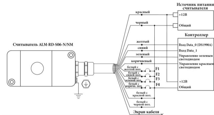
Рисунок 2 – Схема подключения считывателя ALM-RD-S06-N/NM к контроллеру СКУД
