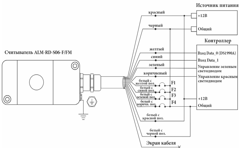
Рисунок 4 – Схема подключения счетчика ALM-RD-S06-F/FM к контроллеру СКУД с питанием счетчика и нагревателя от одного источника питания
