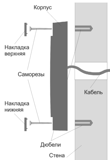
Рисунок 2. Крепление считывателя
