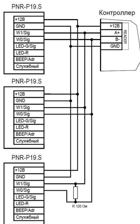
Рисунок 5. Подключение считывателя по интерфейсу OSDP
