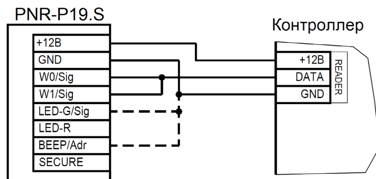
Рисунок 3. Подключение считывателя по интерфейсу Touch Memory
