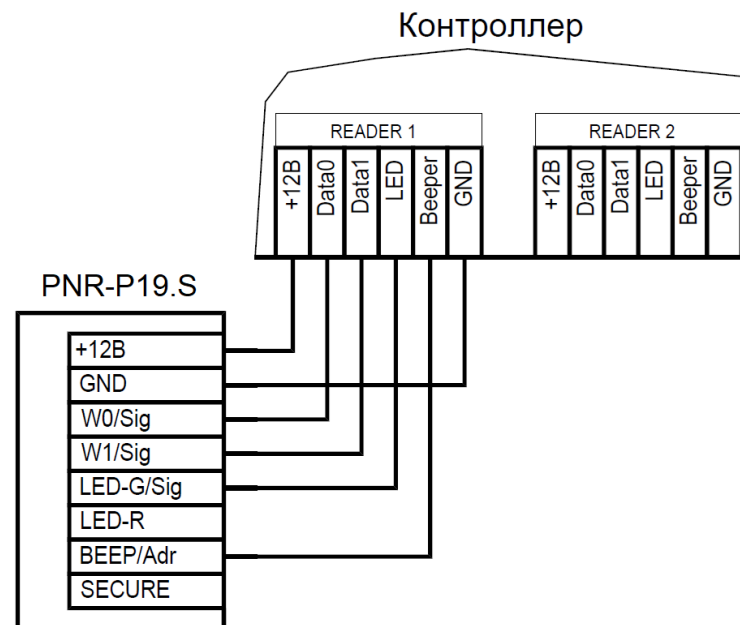
Рисунок 4. Подключение считывателя по интерфейсу Wiegand
