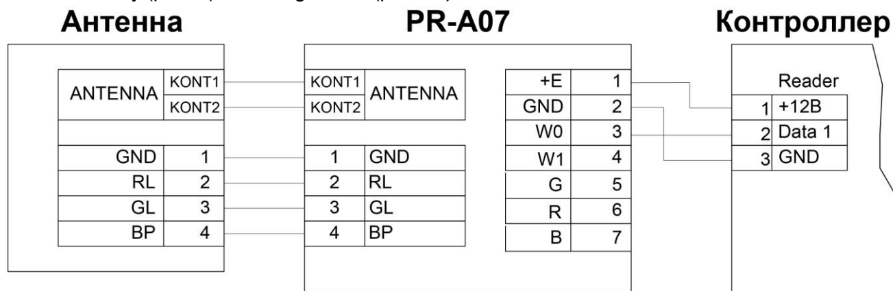
Рисунок 9. Схема подключения считывателя PR-A07 по интерфейсу Touch Memory
