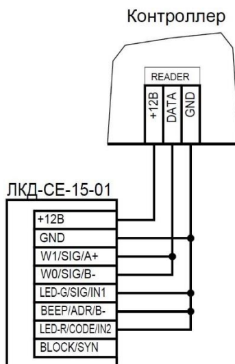
Рисунок 7. Подключение считывателя по интерфейсу Touch Memory
