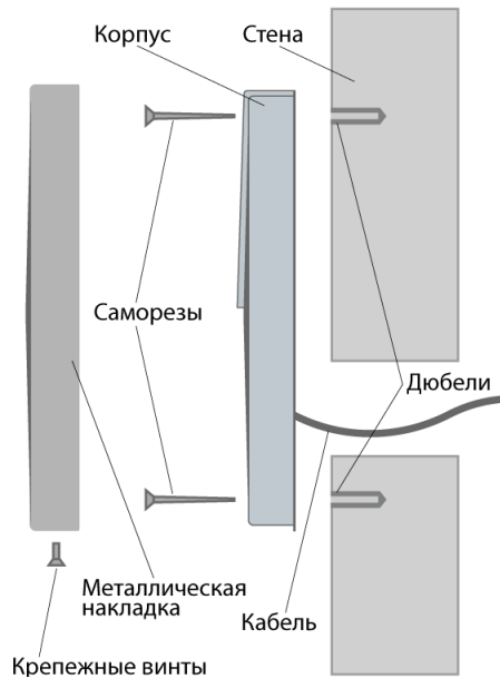
Рисунок 2. Крепление считывателя ЛКД-СЕ-15-01
