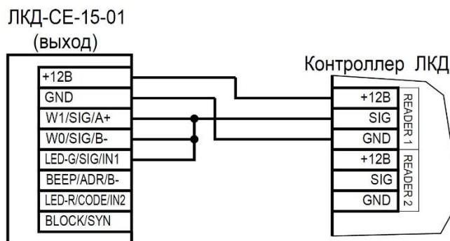
Рисунок 9. Подключение считывателя по интерфейсу ЛКД, адрес 1 (внутренний)
