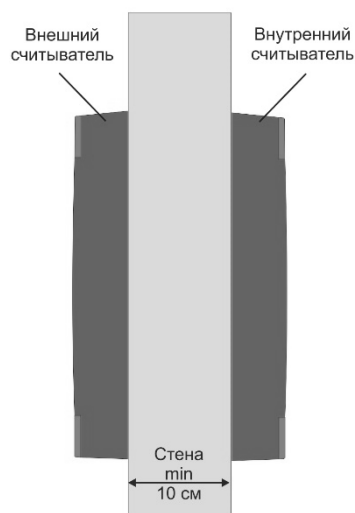
Рисунок 5. Крепление считывателей на одном уровне
