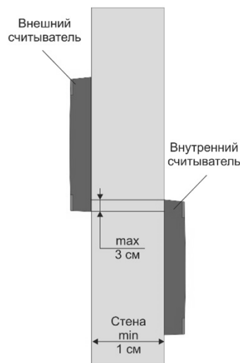
Рисунок 6. Крепление считывателей с разнесением по вертикали
