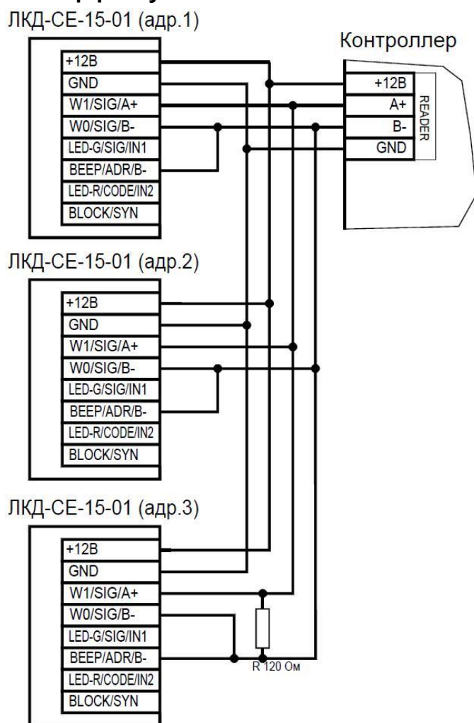
Рисунок 12. Подключение считывателей по интерфейсу OSDP
