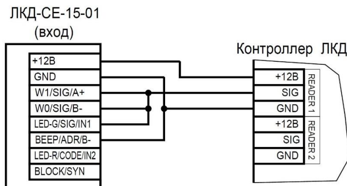
Рисунок 10. Подключение считывателя по интерфейсу ЛКД, адрес 0 (наружный)
