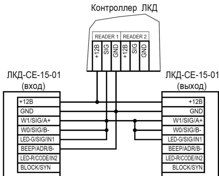
Рисунок 11. Подключение двух считывателей по интерфейсу ЛКД одним кабелем
