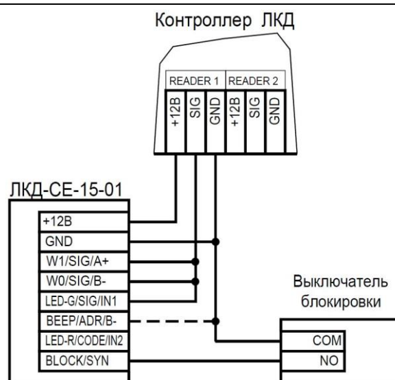
Рисунок 13. Пример подключения провода BLOCK/SYN для ручного включения блокировки
