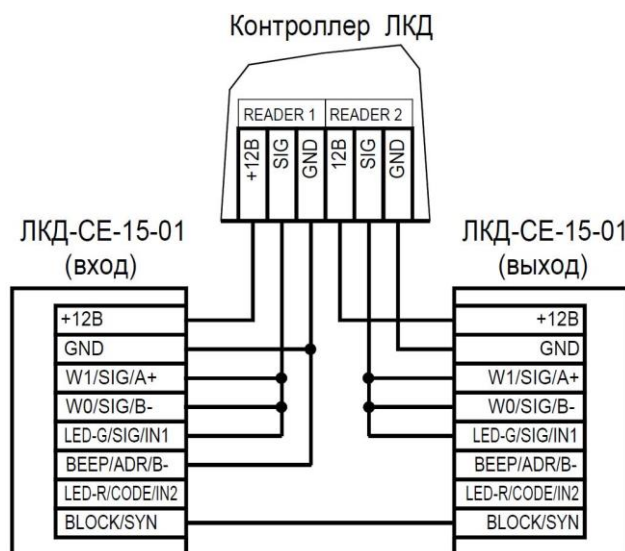
Рисунок 4. Режим синхронизации двух считывателей
