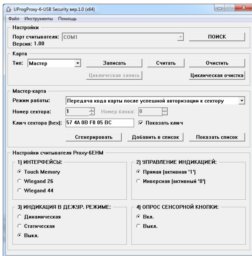
Рис.29 Программирование мастер-карты
