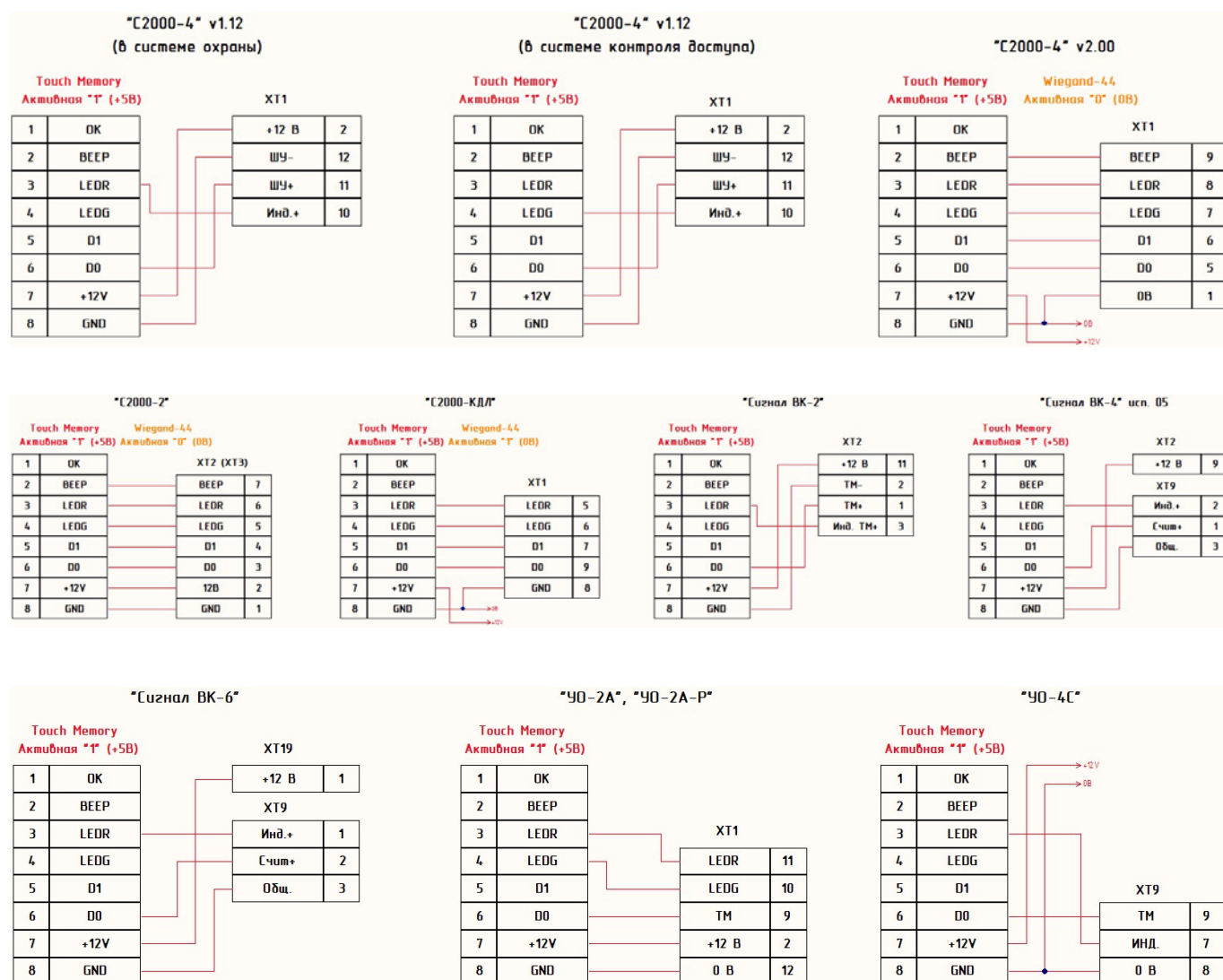
Рис.2.5 Схемы внешних подключений считывателя.
