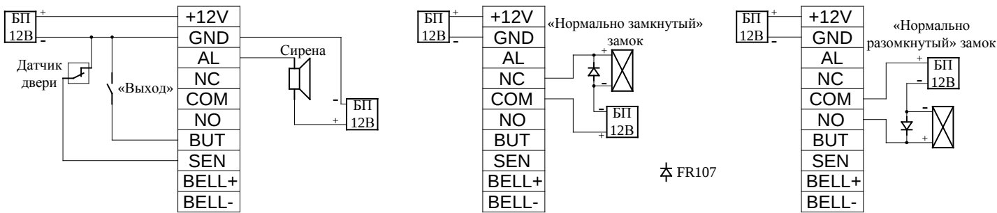
Рисунок 2. Схемы подключения считывателя в автономном режиме
