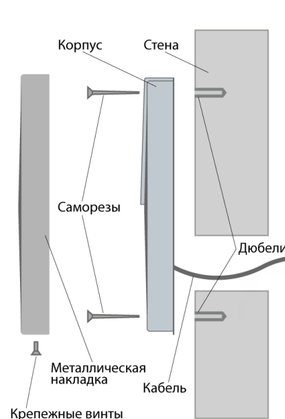
Рисунок 2. Крепление считывателя PNR-P15
