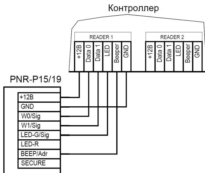
Рисунок 6. Подключение считывателя по интерфейсу Wiegand
