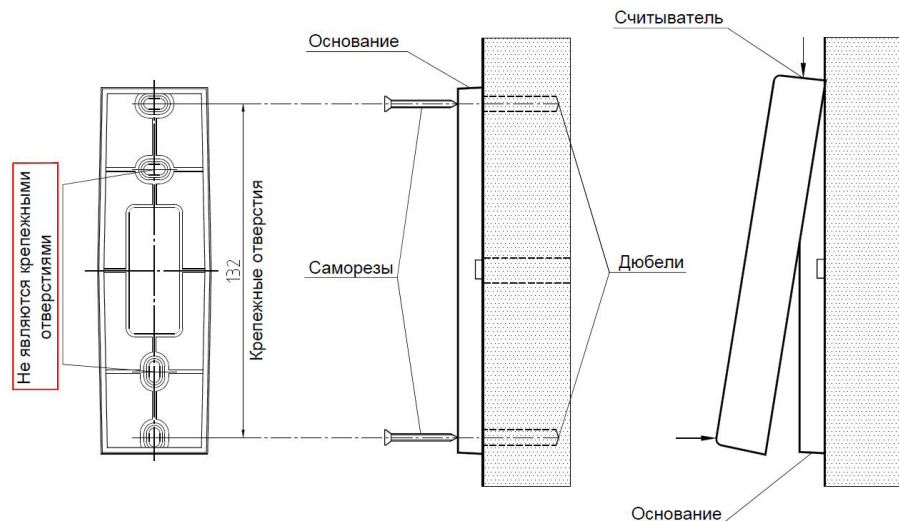
Рисунок 4. Основание
