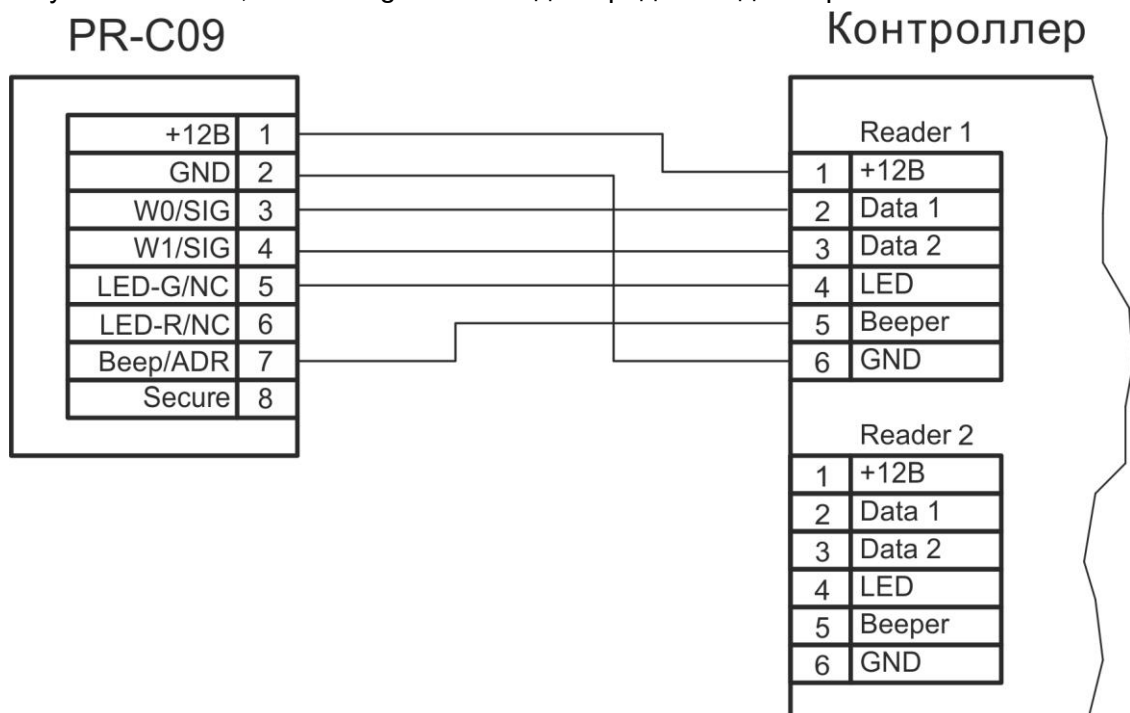
Рисунок 5. Подключение считывателя к разъему контроллера в режиме Wiegand 26
