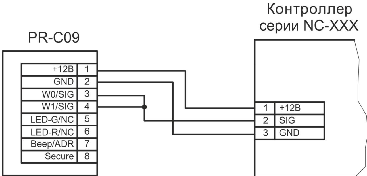
Рисунок 4. Подключение считывателя в режиме Parsec с адресом 1 (внутренний)
