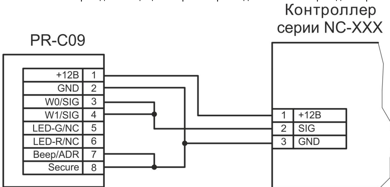
Рисунок 7. Защищенный режим считывателя, подключенного по интерфейсу Parsec с адресом 0
