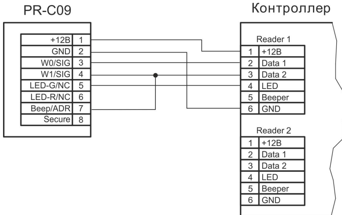
Рисунок 6. Подключение считывателя к разъему контроллера в режиме Wiegand 33
