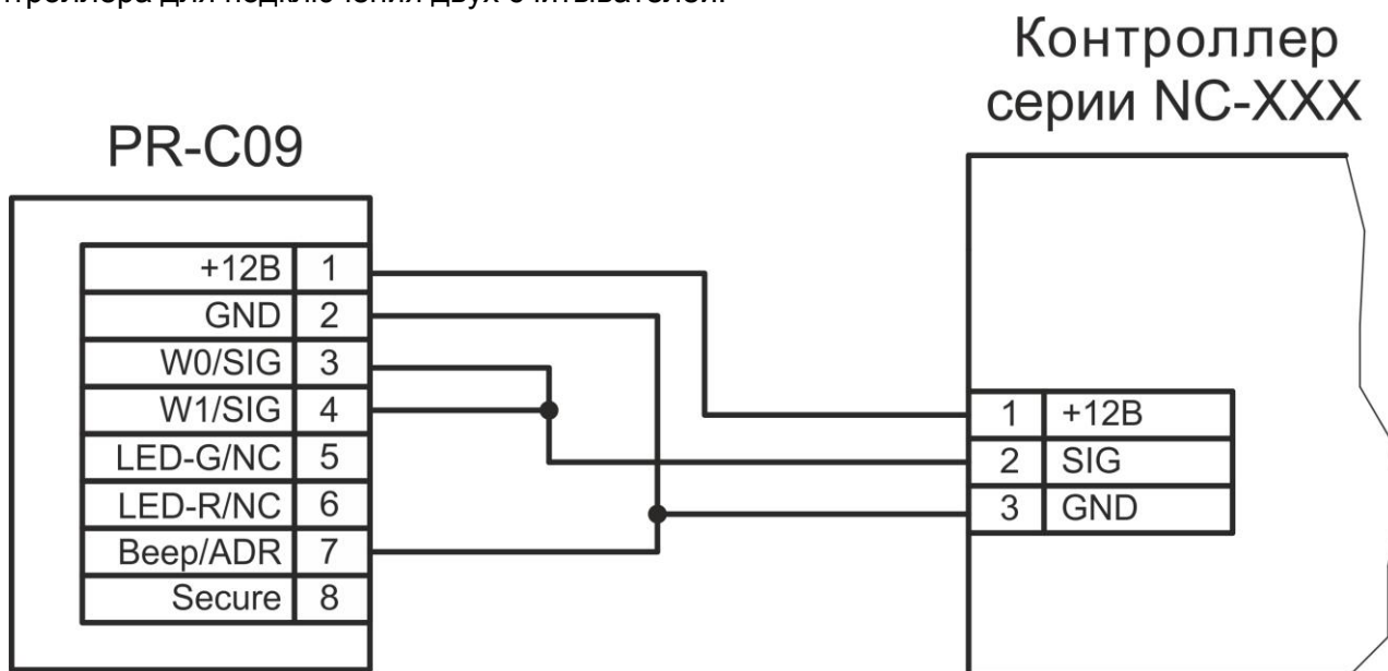
Рисунок 3. Подключение считывателя в режиме Parsec с адресом 0 (наружный)
