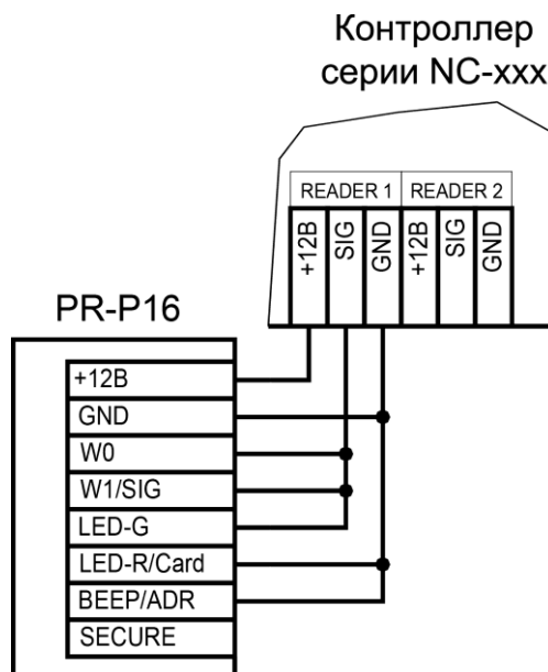
Рисунок 7. Подключение считывателя в режиме Parsec «только карта», адрес 0 (наружный)
