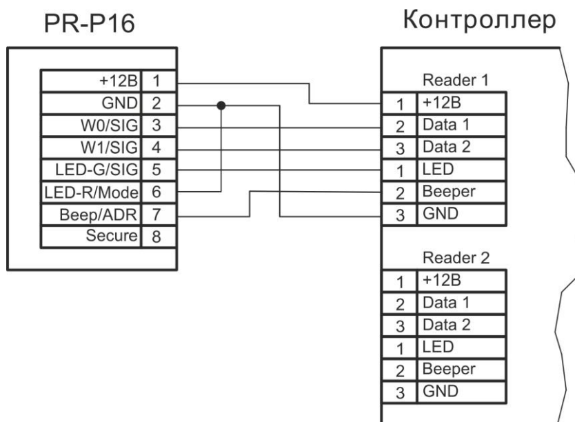
Рисунок 4. Подключение считывателя в режиме Wiegand 26
