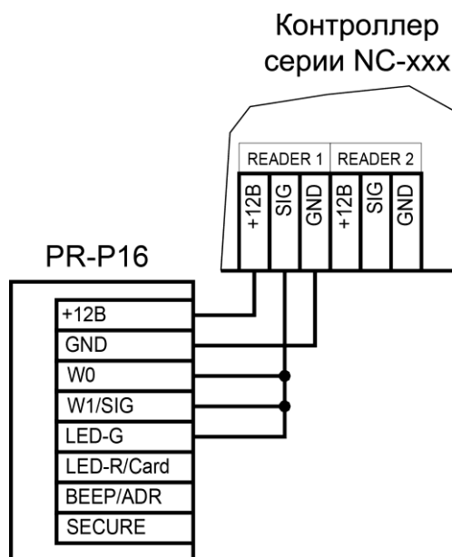
Рисунок 6. Подключение считывателя в режиме Parsec, адрес 1 (внутренний), режим прохода «карта+ПИН»
