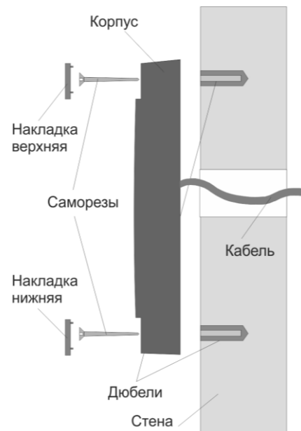
Рисунок 2. Крепление PR-P16
