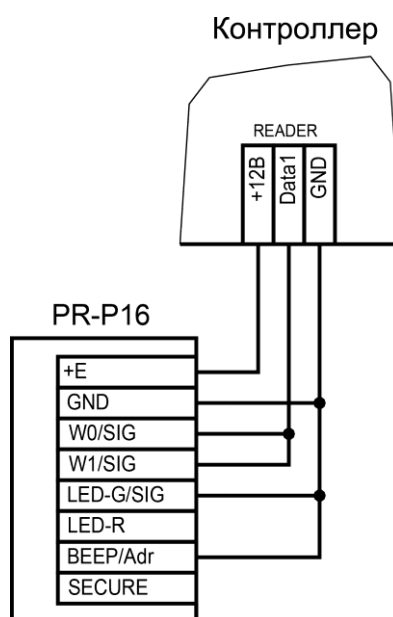
Рисунок 3. Подключение считывателя в режиме Touch Memory
