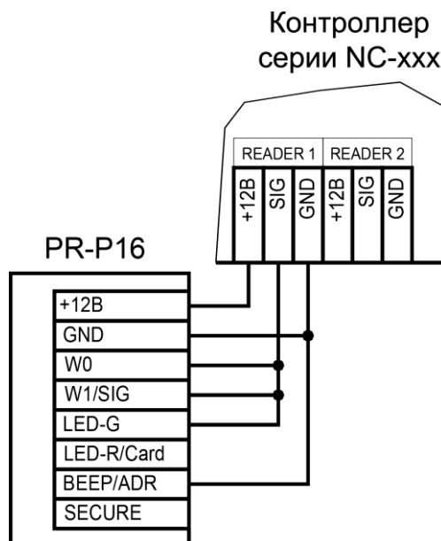
Рисунок 5. Подключение считывателя в режиме Parsec, адрес 0 (наружный), режим прохода «карта+ПИН»
