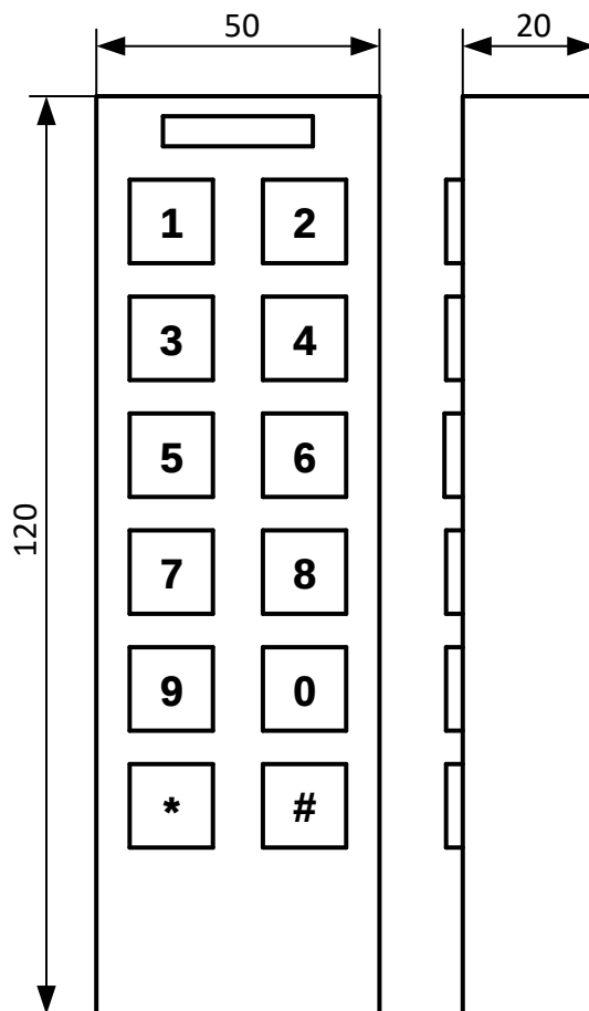
Рисунок 1. Внешний вид и габаритные размеры считывателя
