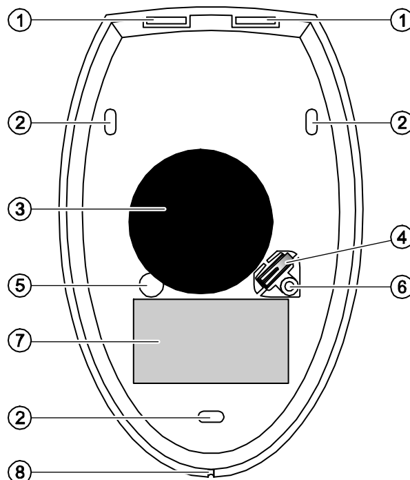
Рис. 1. Вид основания корпуса оповещателя.
