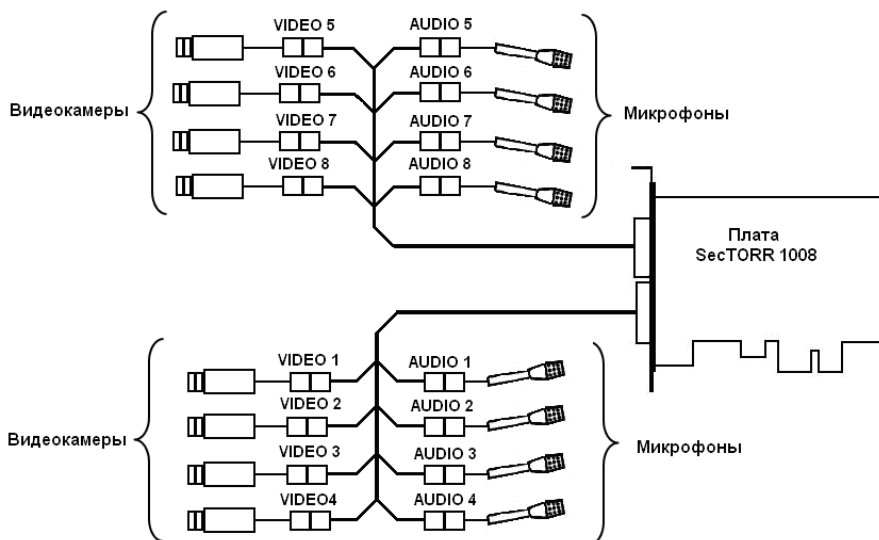
Рисунок 3 – Схема подключения видеокамер
