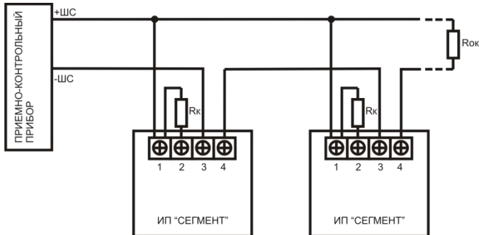
Рис.1. - Типовая схема включения извещателя ИП 435-4-Ex «Сегмент» к ПКП с однополярным шлейфом сигнализации. Величина резисторов Rk и Rok определяется в соответствии с техническим описанием ПКП.
