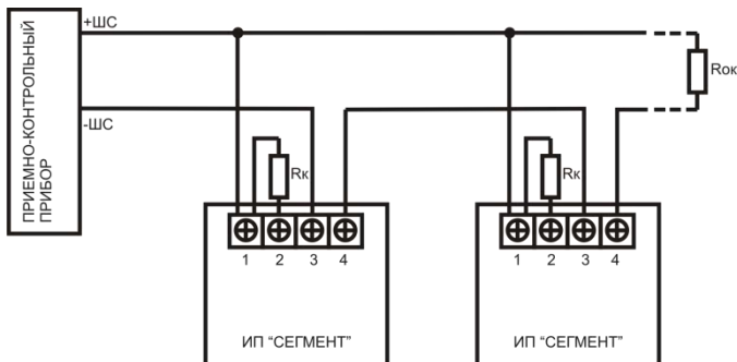
Рис.1. - Типовая схема включения извещателя ИП 435-4-Ex «Сегмент» к ПКП с однополярным шлейфом сигнализации. Величина резисторов Rk и Rок определяется в соответствии с техническим описанием ПКП.
