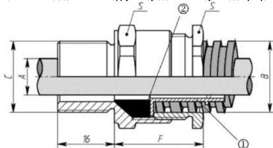
Рис. 1 – Вариант герметичного кабельного ввода универсального взрывозащищенного.
