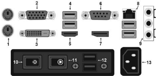
Рисунок 2. Назначение интерфейсов системного блока.
