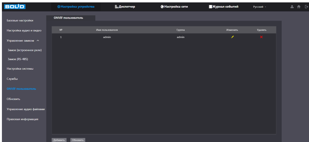
Рисунок 8.9 – Интерфейс просмотра учётной записи ONVIF пользователя
