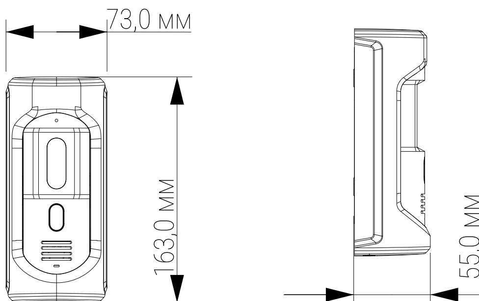
Рисунок 4.1 – Габаритные размеры
