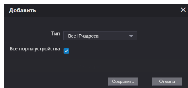
Рисунок 10.18 – Добавить «Все IP-адреса»
