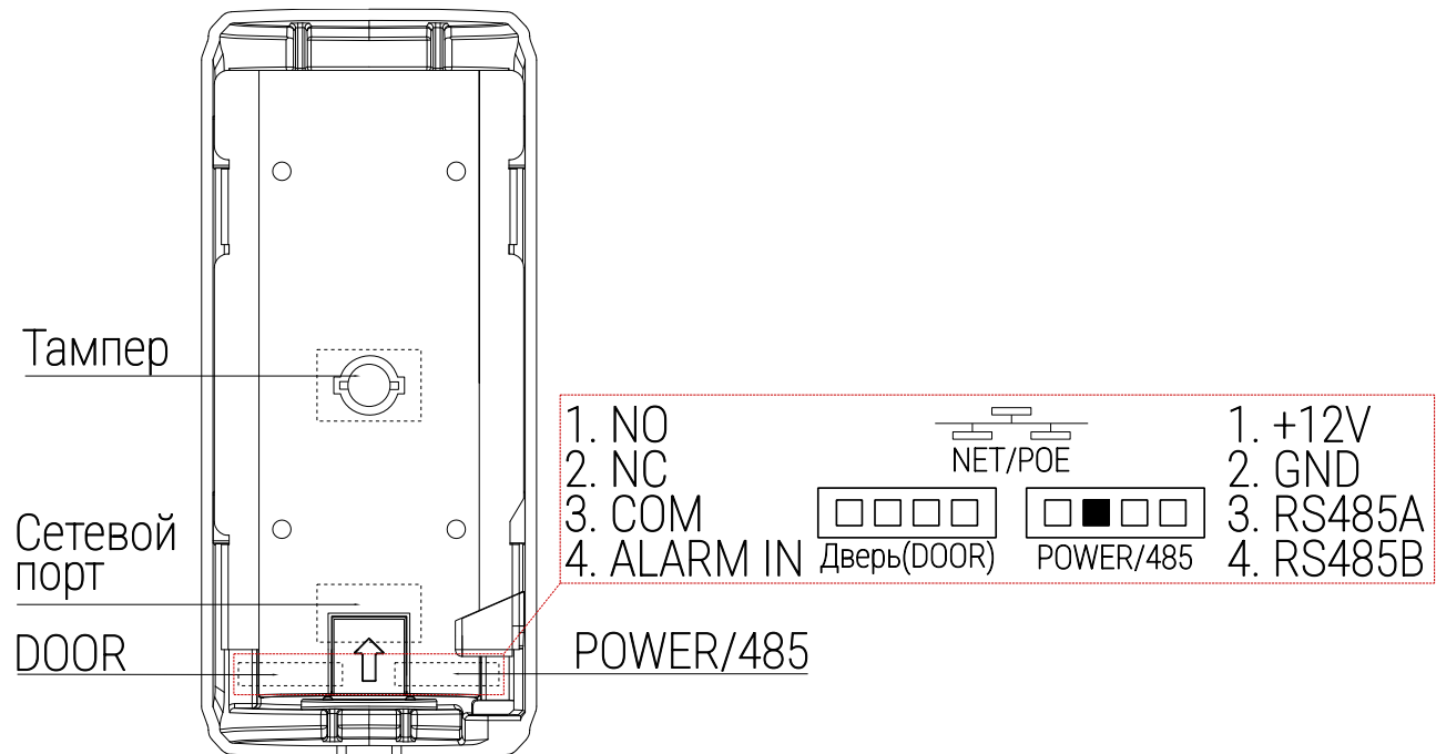
Рисунок 3.2 – Задняя панель корпуса
