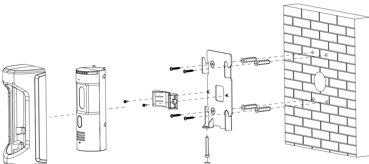
Рисунок 4.3 – Схема крепления
