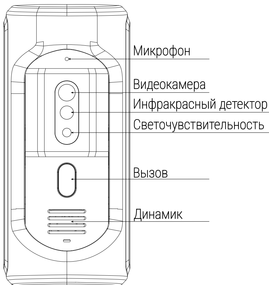
Рисунок 3.1 – Передняя панель
