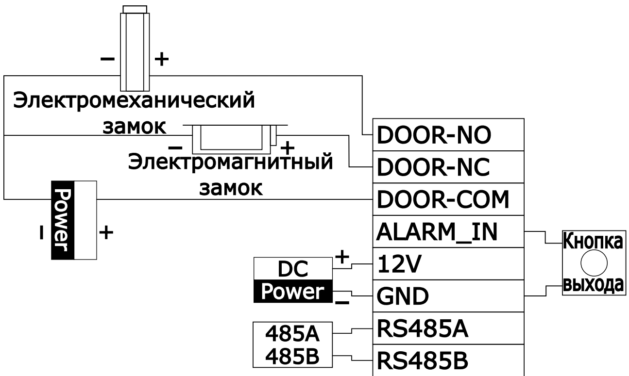
Рисунок 3.4 – Схема подключения. Замок 1
