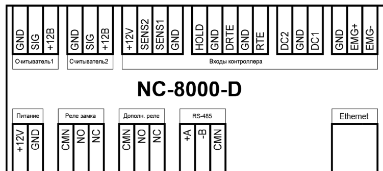
Рисунок 2. Схема платы контроллера
