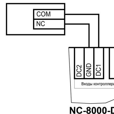
Рисунок 15. Схема подключения дверного контакта
