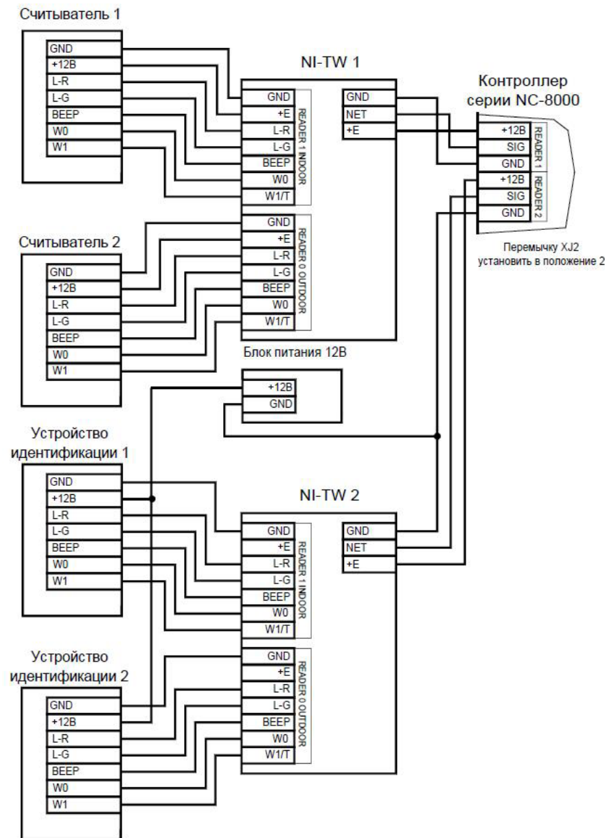
Рисунок 5. Схема подключения 2 считывателей и 2 устройств идентификации с интерфейсом Wiegand
