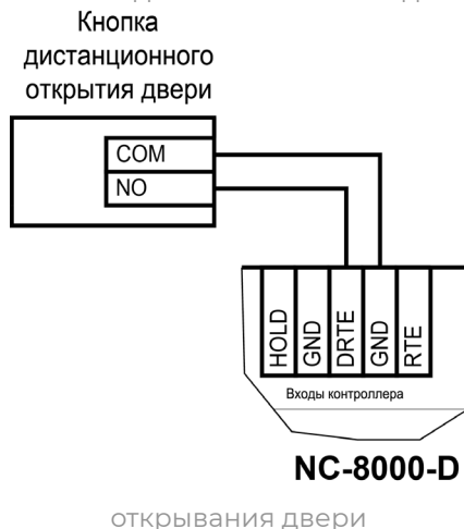
Рисунок 14. Схема подключения кнопки дистанционного
