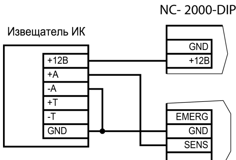
Рисунок 14. Подключение охранного датчика без контроля подводящих проводов
