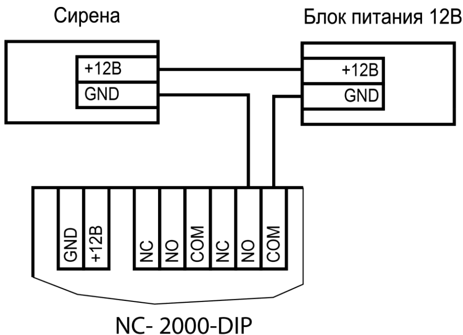
Рисунок 16. Подключение сирены к дополнительному реле
