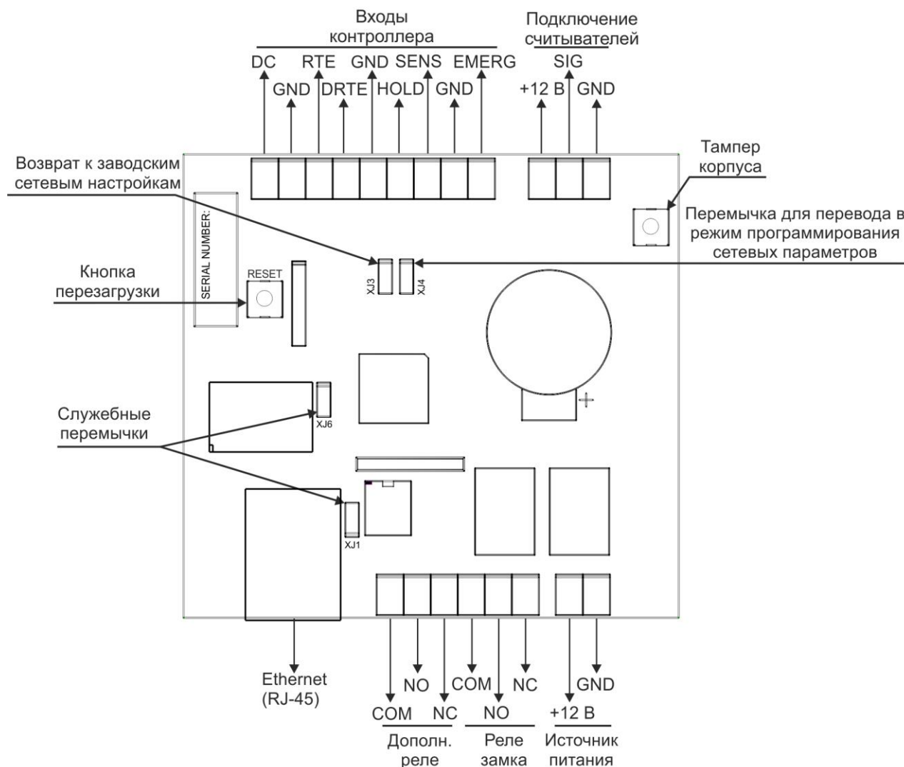
Рисунок 2. Схема платы контроллеров NC-2000-DIP
