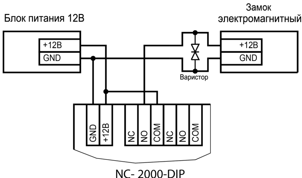
Рисунок 8. Питание замка от того же источника, что и контроллер
