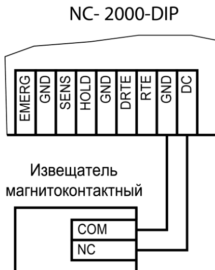
Рисунок 12. Схема подключения DC без контроля подводящих проводов
