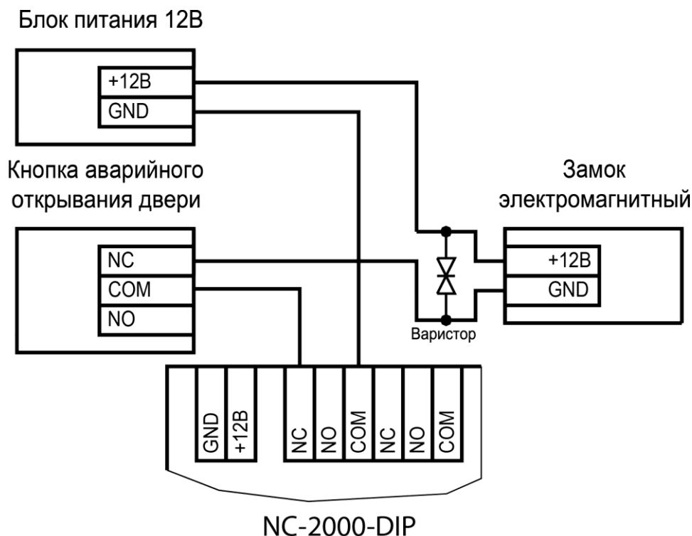
Рисунок 7. Подключение запираемых напряжением замков к контроллеру с аварийной кнопкой
