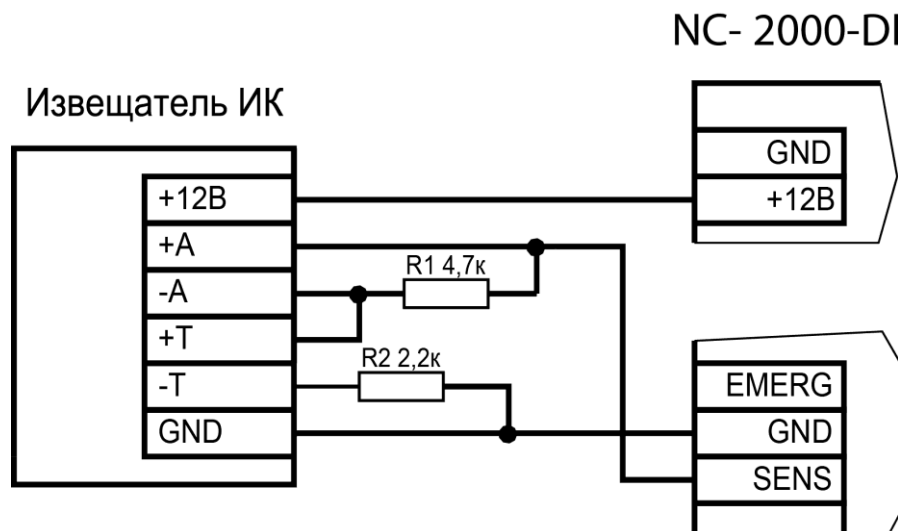
Рисунок 15. Подключение охранного датчика с контролем подводящих проводов
