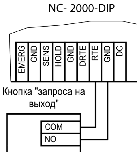
Рисунок 10. Схема подключения кнопки запроса на выход
