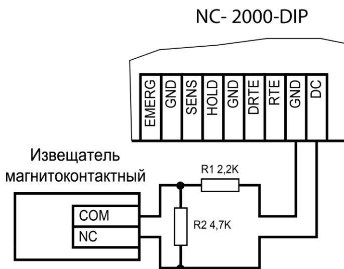
Рисунок 13. Схема подключения DC с контролем подводящих проводов
