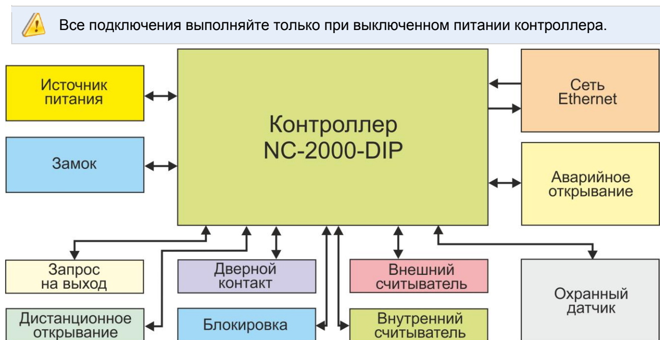
Рисунок 4. Оборудование, подключаемое к контроллеру NC-2000-DIP
