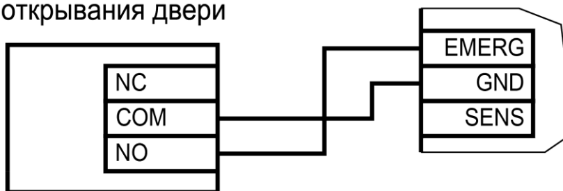
Рисунок 18. Подключение кнопки аварийного выхода к одному контроллеру
