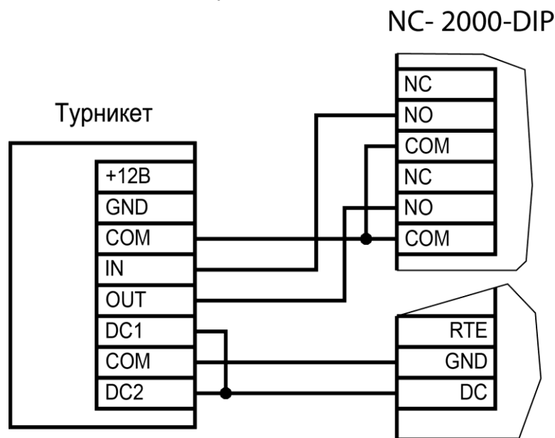
Рисунок 9. Схема подключения турникета с нормально разомкнутыми контактами к контроллеру
