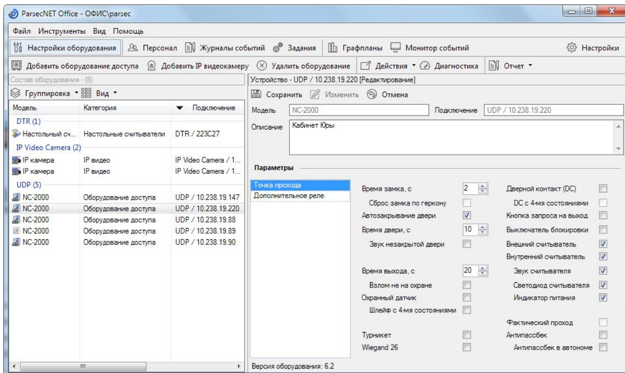
Рисунок 24. Настройка контроллера в ParsecNET 3
