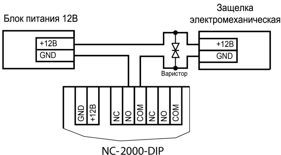
Рисунок 6. Схема подключения отпираемых напряжением замков к контроллеру
