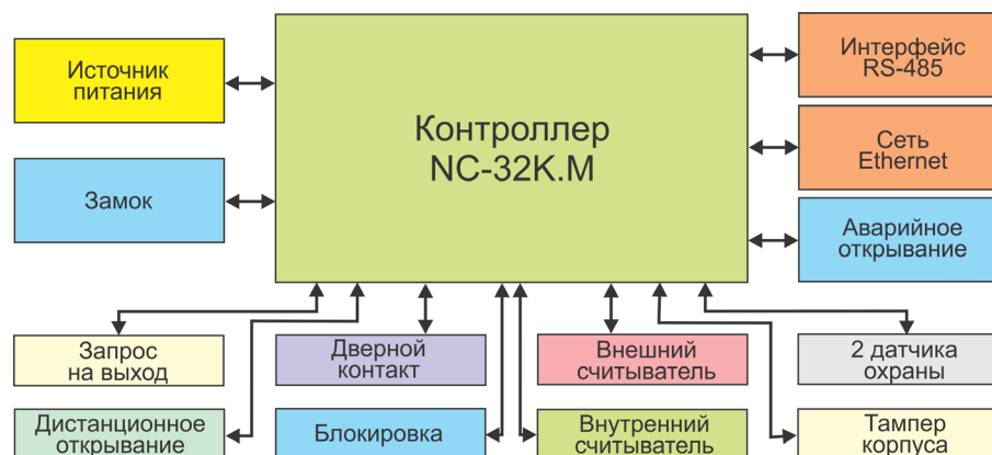
Рисунок 7. Оборудование, подключаемое к контроллеру NC-100K-IP
