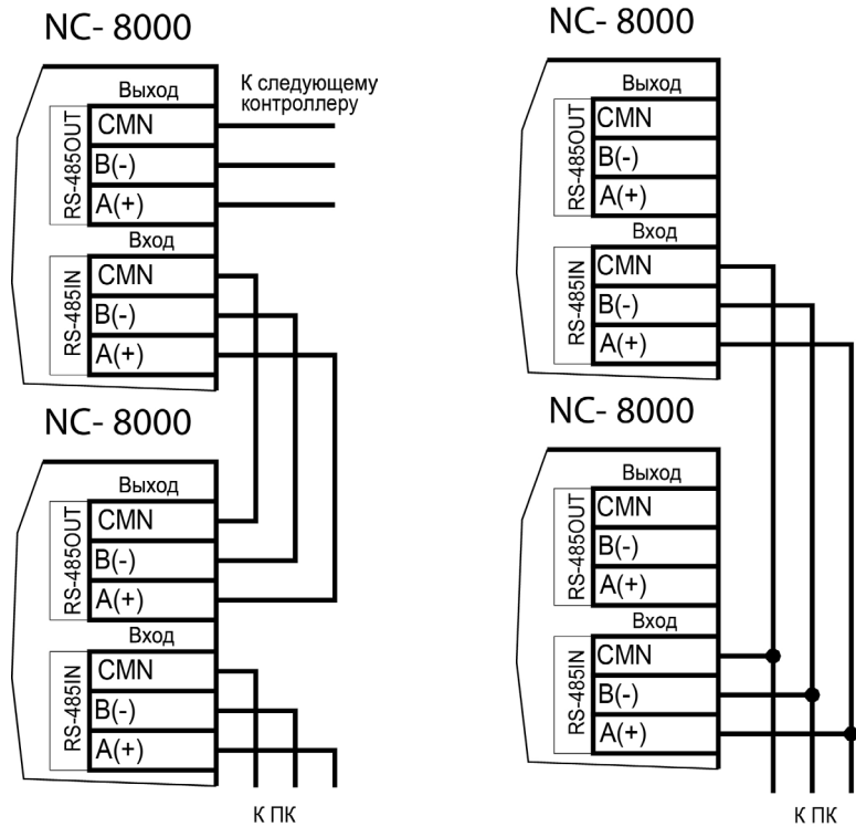
Рисунок 28. Схема соединения контроллеров по топологии «Шина»
