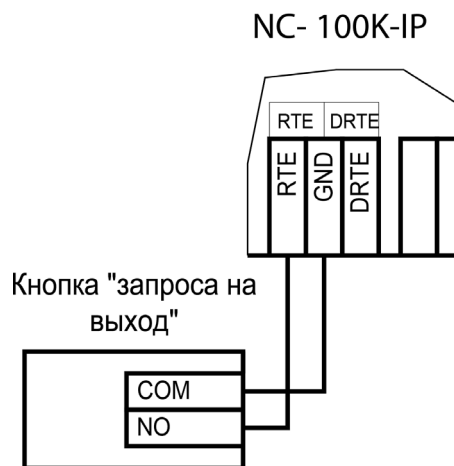
Рисунок 18. Схема подключения кнопки запроса на выход
