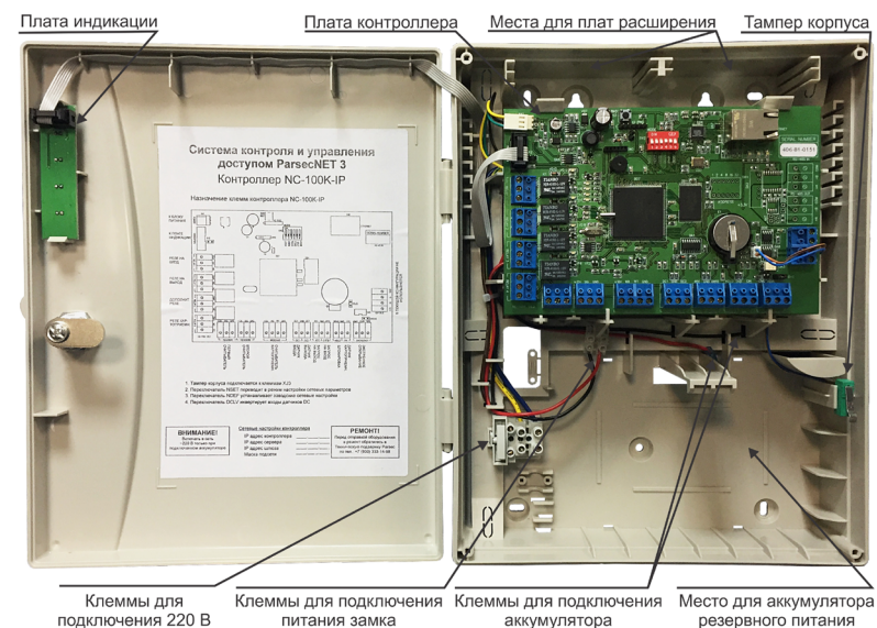
Рисунок 1. Открытый корпус с платой контроллера
