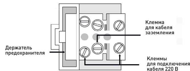
Рисунок 6. Клеммная колодка для кабеля питания
