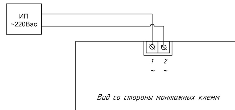
Схема подключения светового табло «Сфера Премиум 220В»
