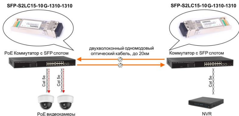
Рис.4 Типовая схема подключения модулей SFP-S2LC15-10G-1310-1310
