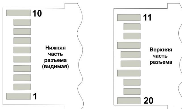
Рис.3 Распиновка SFP+ разъема
