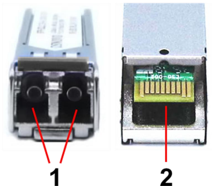
Рис.2 SFP+ модули SFP-S2LC15-10G-1310-1310 и SFP-M2LC05-10G-850-850, разъемы спереди/сзади.
