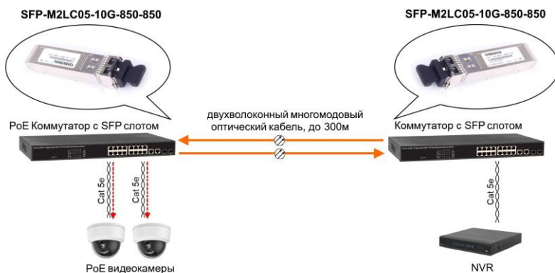
Рис.5 Типовая схема подключения модулей SFP-M2LC05-10G-850-850
