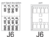
Рисунок 22 – Контакты порта RS485
