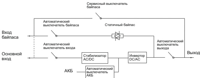
Рисунок 10 – Структура ИБП
