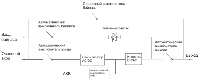
Рисунок 18 – Структура ИБП
