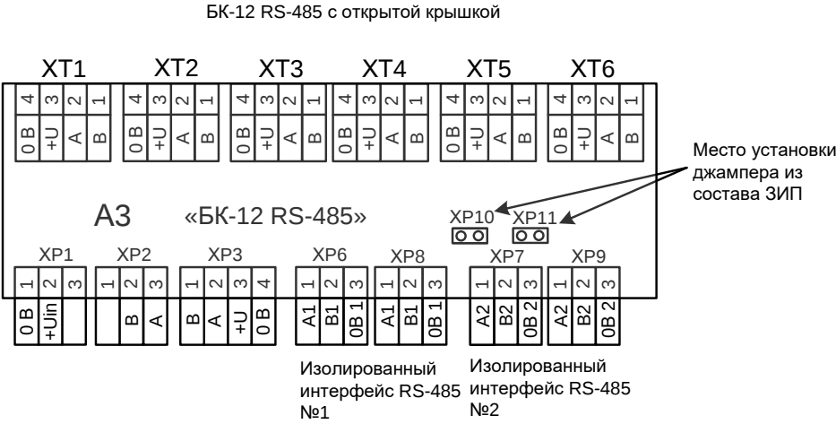
Рис.3 Схематичное изображение разъемов на плате БК-12 RS485, крышка открыта.
