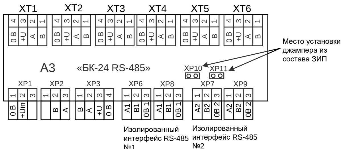
Рис.3 Схематичное изображение разъёмов на плате БК-24 RS485, крышка открыта.
