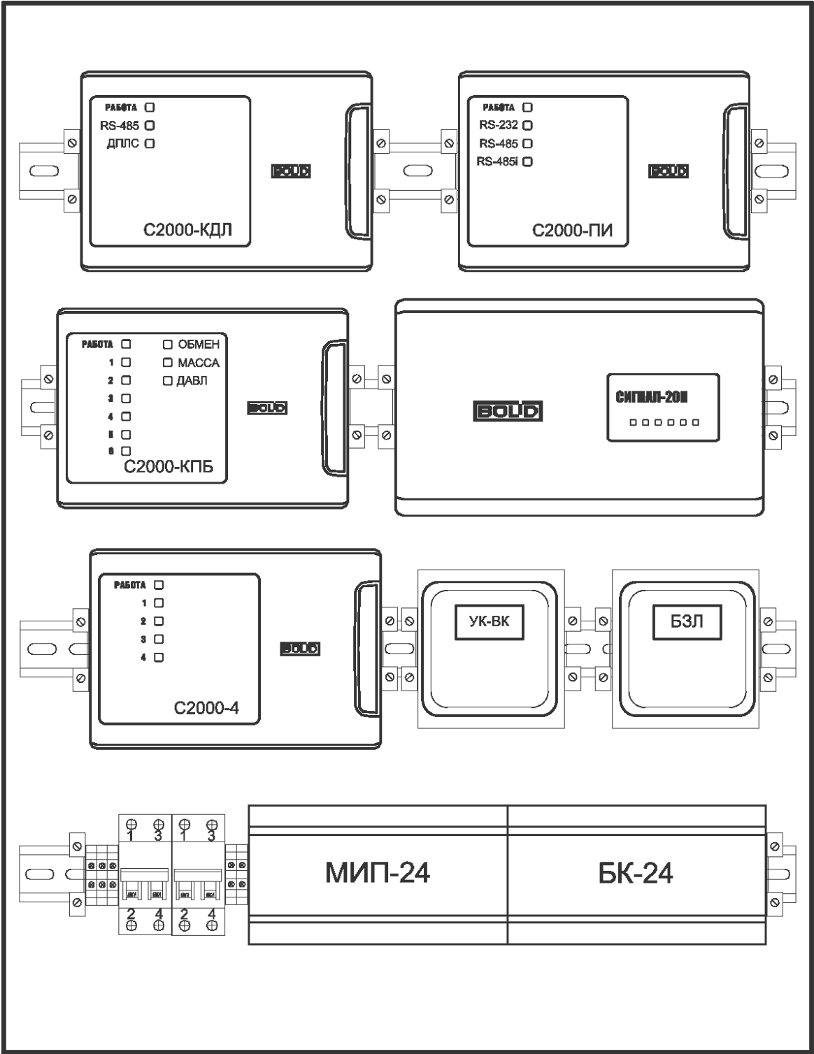
Пример №2 компоновки оборудования в ШПС-24
