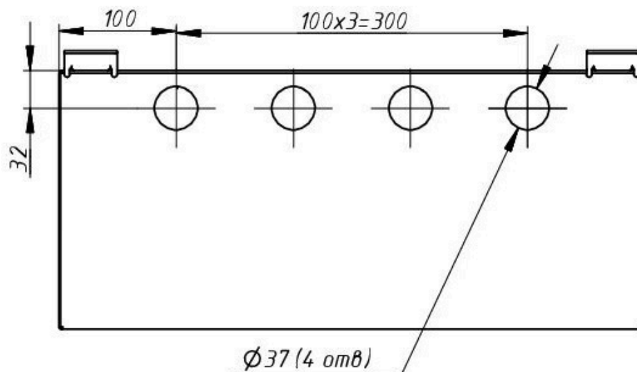
Вид корпуса сверху
