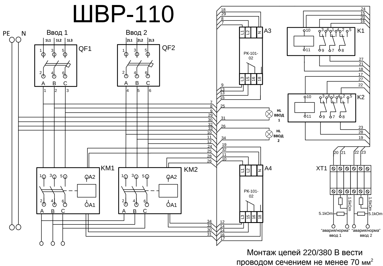
Рисунок 3. Схема внутренних соединений ШВР-110.
