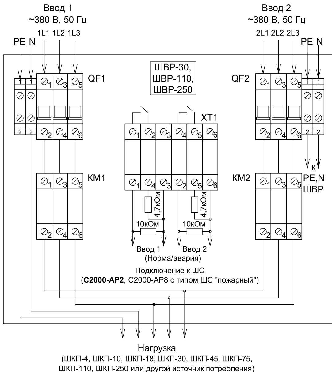
Рисунок 2. Возможность применения ШВП в адресной системе
