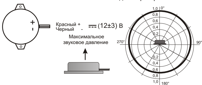
Рис.2 Схема подключения и диаграмма направленности оповещателя ПКИ-МШ.
